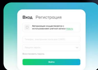
Страница авторизации
